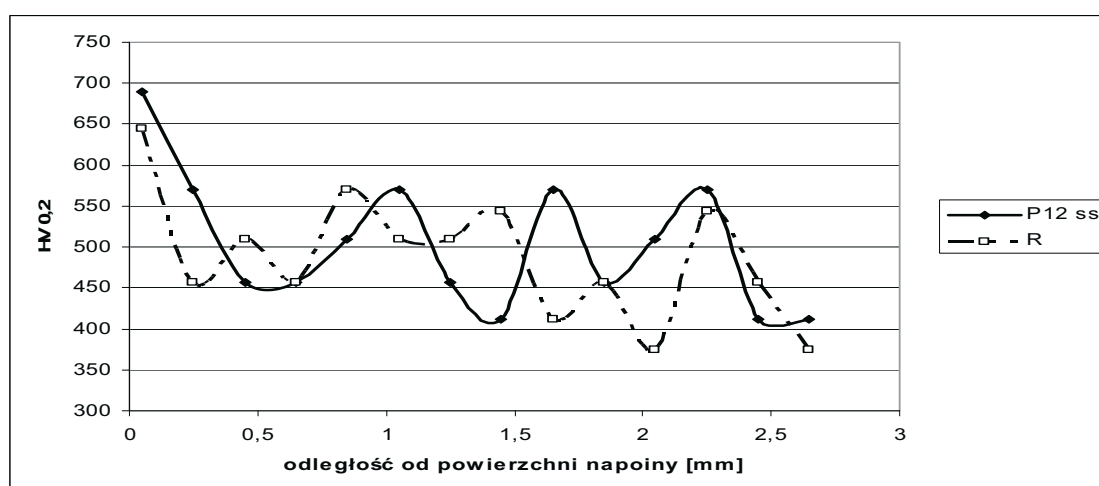
Rys. 5. Mikrotwardość napoiny po korozji w spalinach: P12ss – próbka ekspozowana w komorze, zawór pracujący w silniku okrętowym
