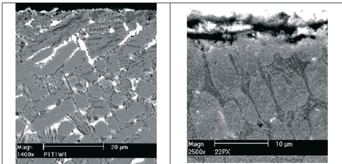
Fot. 3. Mikrostruktura na przekroju napawanej przylgni zaworu zaworu napawanego po ekspozycji w komorze; Zgląd trawiony SEM/EDS
