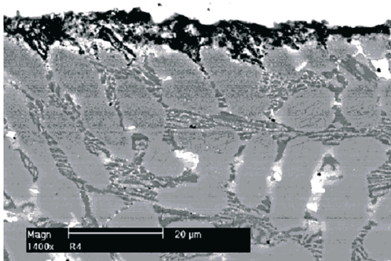
Fot. 4. Mikrostruktura na przekroju napawanej przylgni zaworu zaworu po ekspozycji w komorze; Zgląd trawiony SEM/EDS
