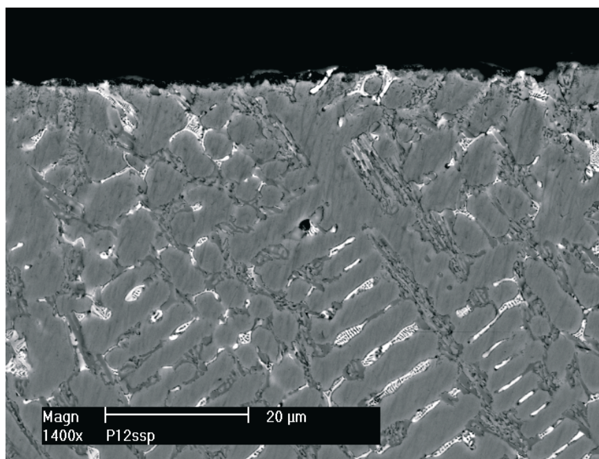
Fot. 2. Mikrostruktura napoiny na powierzchni przylgni
