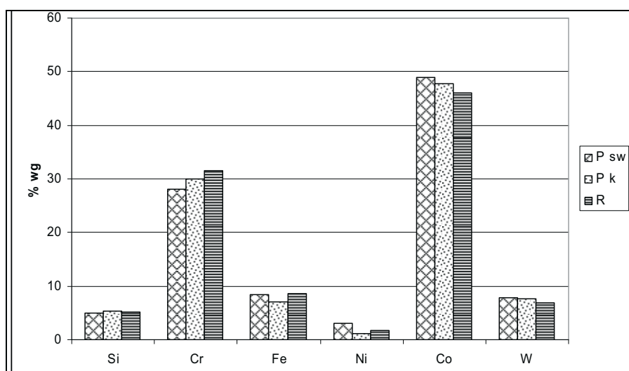
Rys. 4. Analizy chemiczne w mikroobszarach przy powierzchni napoiny; Psw - warstwa napoiny zaworu badanego w komorze w stanie wyjściowym, Pk - na poina na przyłgni zaworu poddanego korozji w komorze, R - napoina na przyłgni zaworu eksploatowanego na statku
